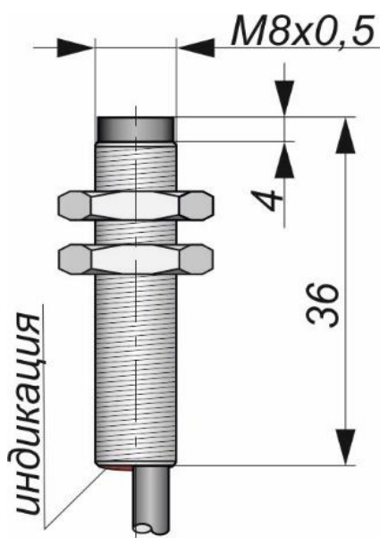
Габаритный чертеж
