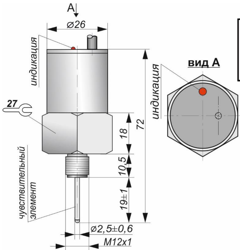
Габаритный чертеж
