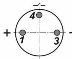
Цоколевка разъема
