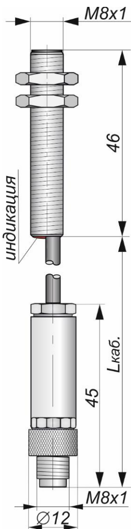
Габаритный чертеж
