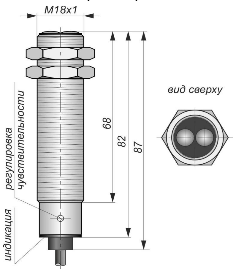
Габаритный чертеж
