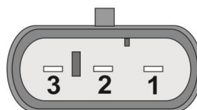
Цоколевка разъема
