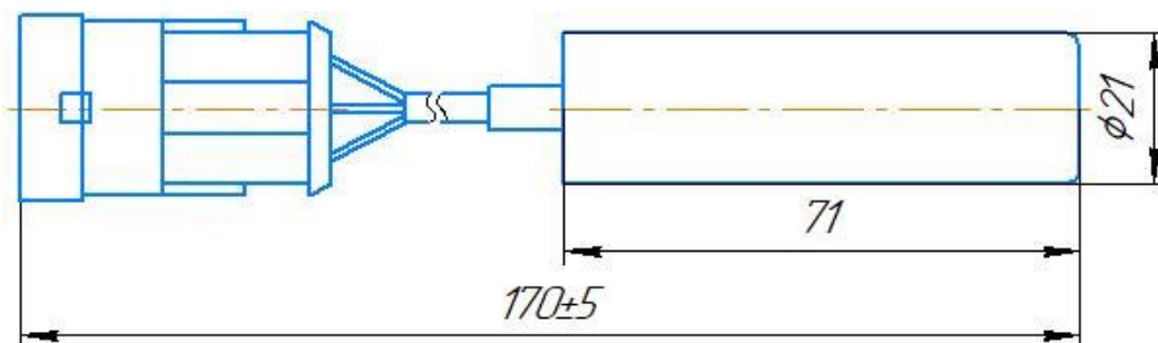
Нормально-разомкнутый контакт
