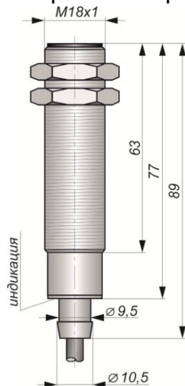
Габаритный чертеж
