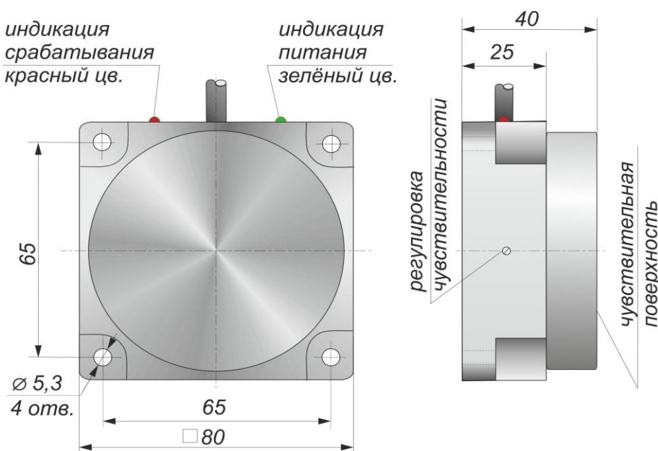
Габаритный чертеж
