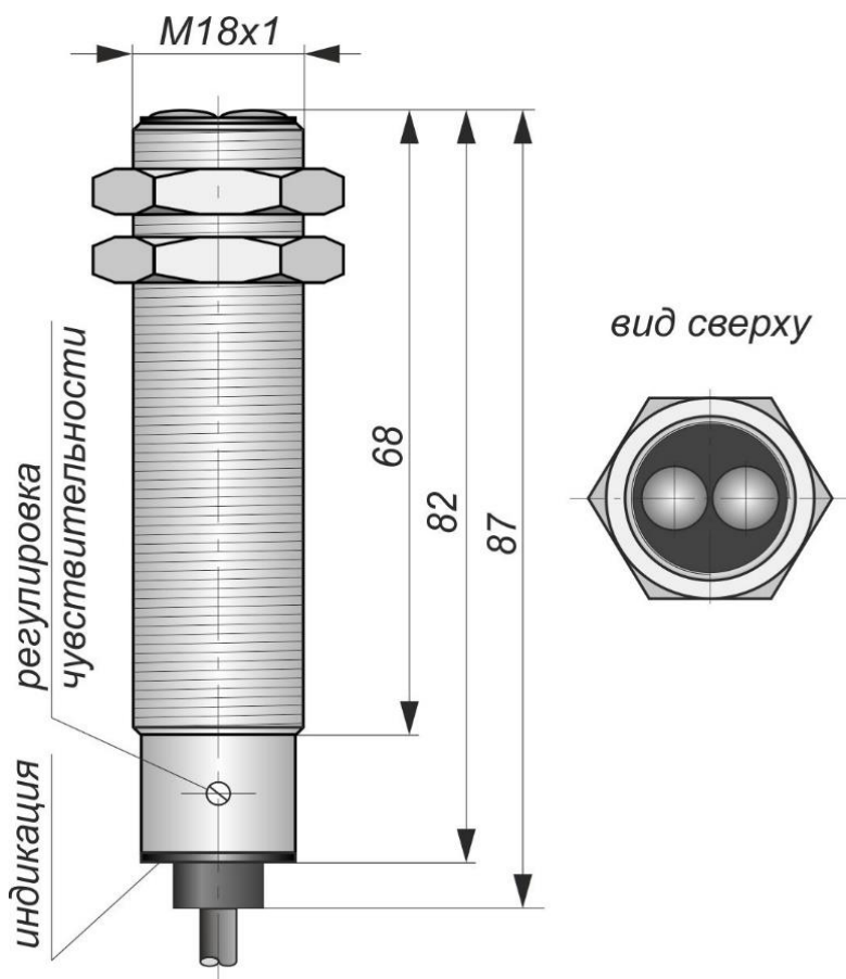
Габаритный чертеж
